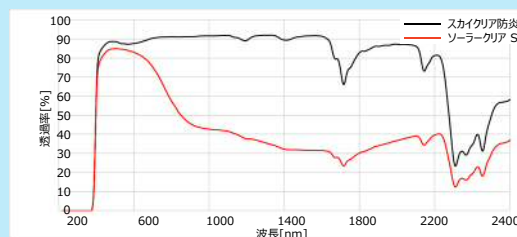
全光線透過率グラフ
